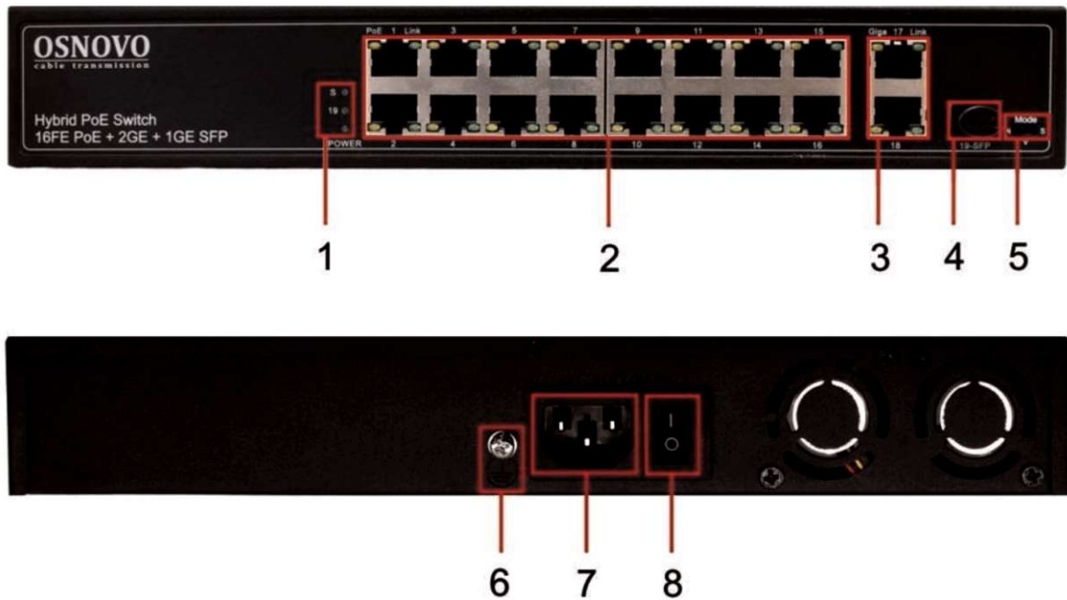
Рис. 3 Панели подключения коммутатора SW-61621(300W)
