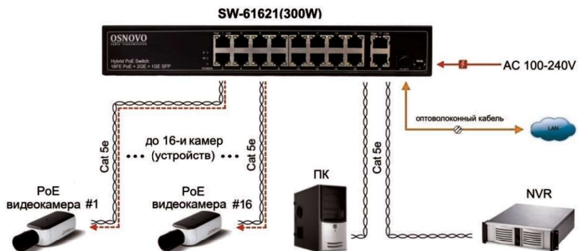
Рис.4 Типовая схема подключения коммутатора SW-61621(300W)
