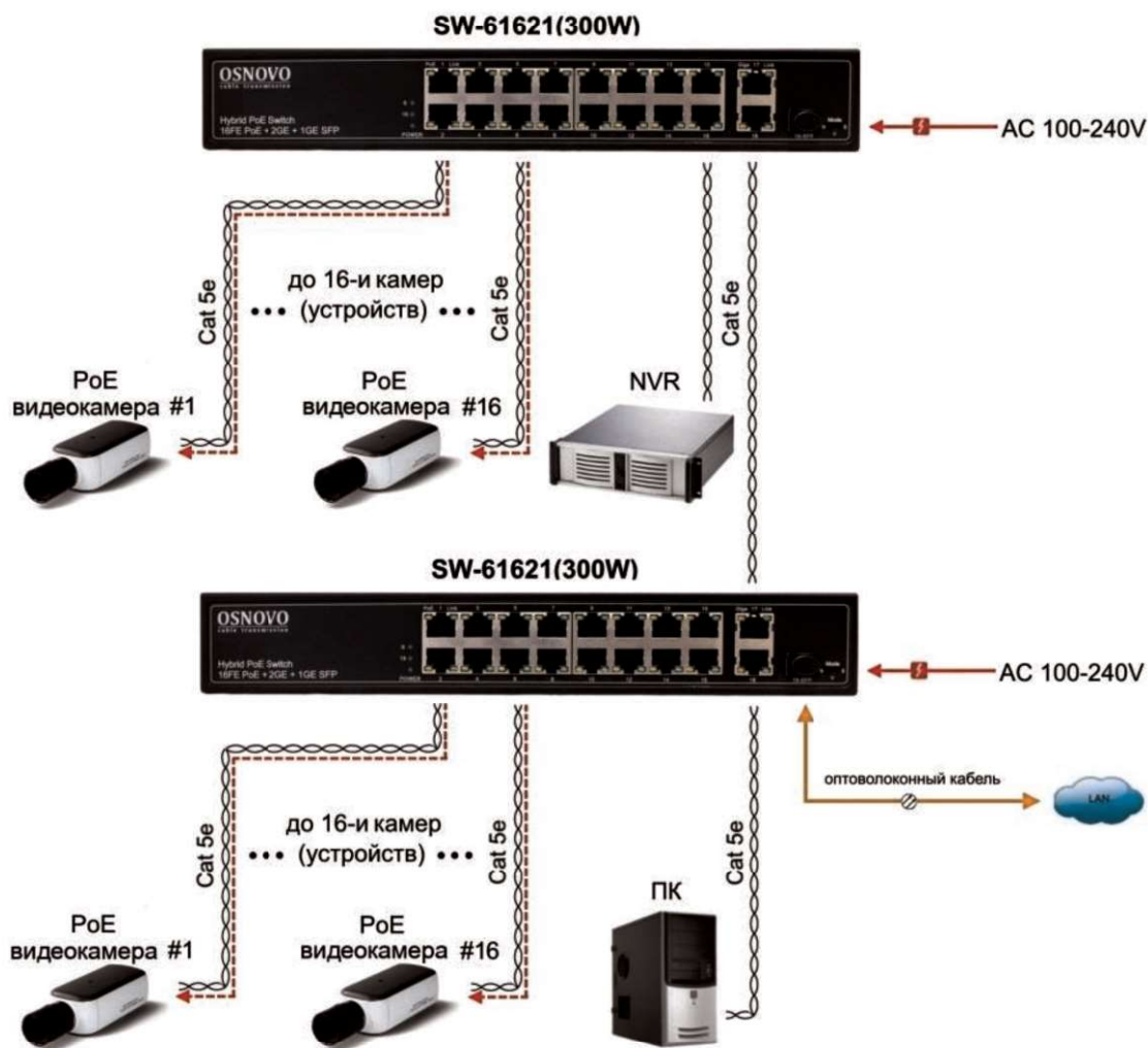
Рис.5 Схема каскадного подключения коммутатора SW-61621(300W)
