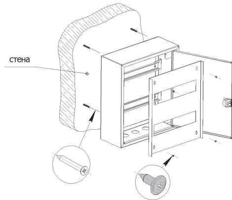
Рис.1. Схема монтажа
