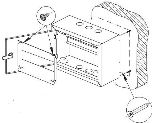
Рис.1. Схема монтажа
