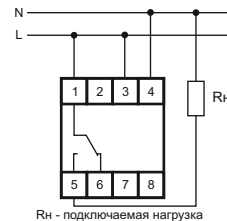
Рн - подключаемая нагрузка Схема подключения изделия и нагрузки к сети 230В.
