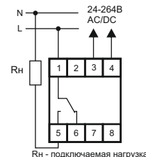
Рн - подключаемая нагрузка Схема подключения изделия и нагрузки, питающихся от разных источников питания.
