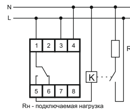
Рн - подключаемая нагрузка Схема подключения изделия с использованием контактора ток нагрузки более 16А.
