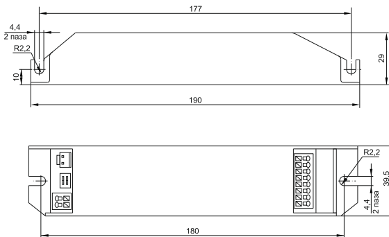
Рисунок 1 – Конвертер БАП200-1,0(3,0)
