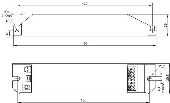
Рисунок 1 – Конвертер БАП200-1,0(3,0)
